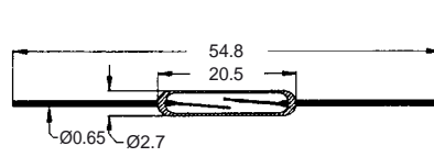
K-236. kép REED 2 méretei
