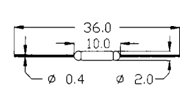
K-237. kép REED 4 méretei
